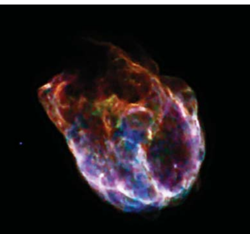
钱德勒X光天文台拍摄到巨大星体解体后的残骸
